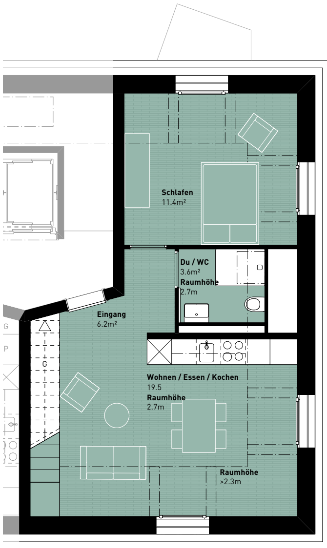
Grundriss
