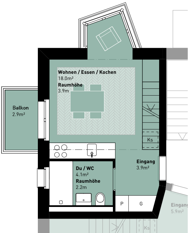
Grundriss
