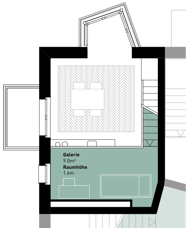
Grundriss Galerie
