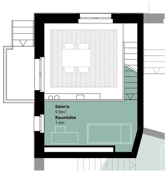
Grundriss Galerie
