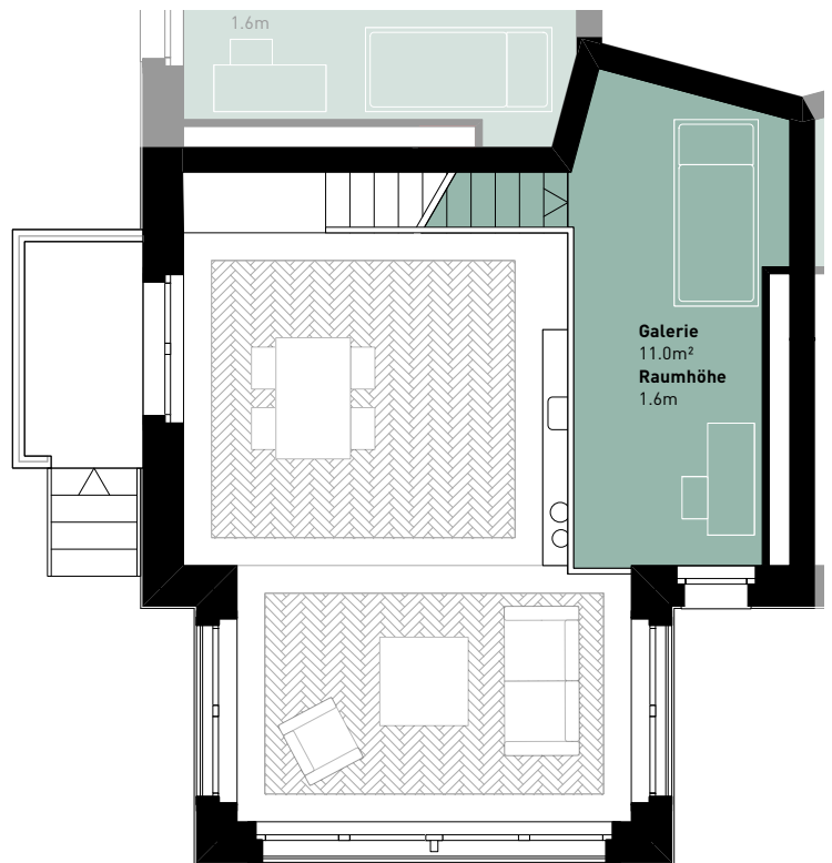
Grundriss Galerie
