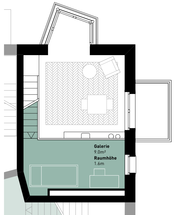
Grundriss Galerie
