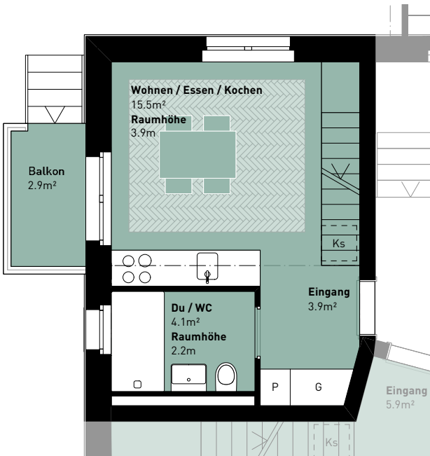
Grundriss
