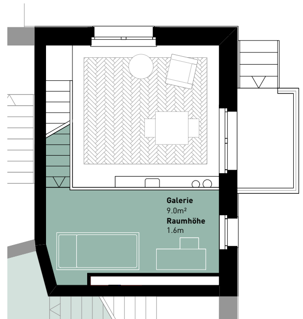
Grundriss Galerie
