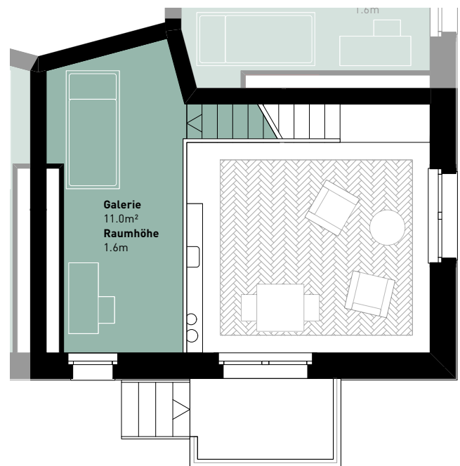
Grundriss Galerie
