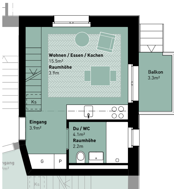
Grundriss
