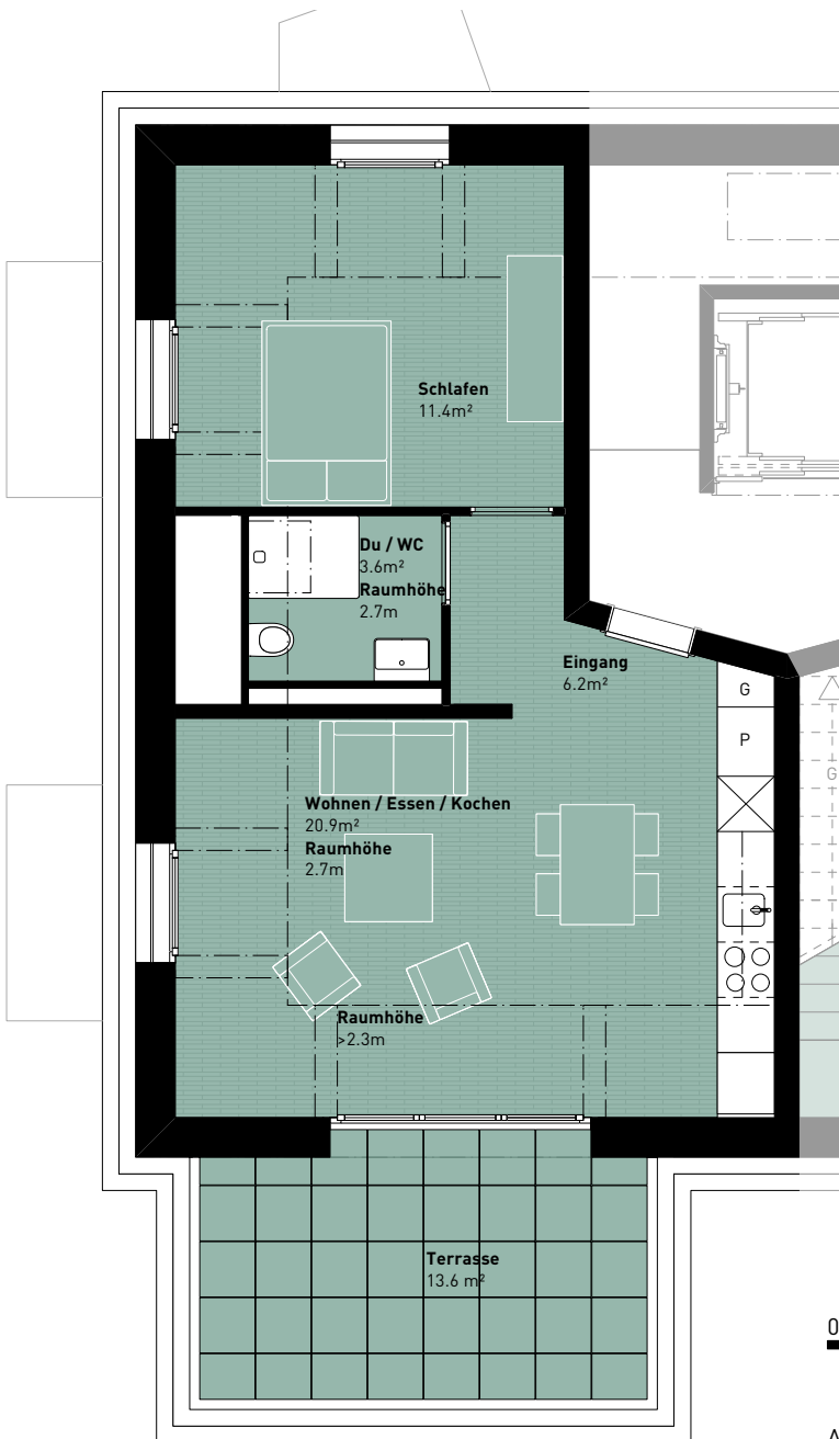
Grundriss
